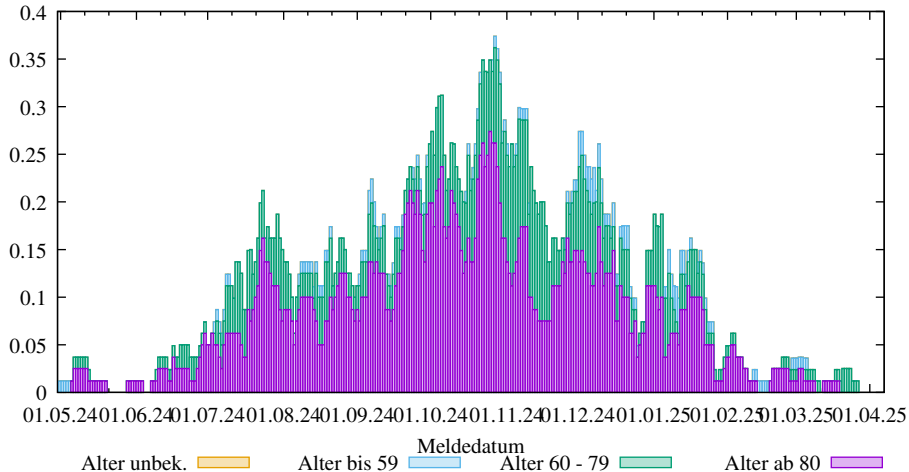
Rel. 7-Tage-Summe der neuen COVID-19 Verstorbenen in Niedersachsen (2025-04-28/Short, D. Lippold, https://covid19-de-stats.sourceforge.io/ Lizenz: CC BY-ND 4.0, Daten: Robert Koch-Institut (RKI), dl-de/by-2-0)
