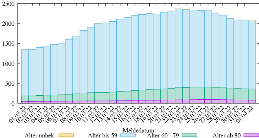
Rel. 7-Tage-Summe der neuen COVID-19 Infizierten in Thüringen (2025-03-09/2203, D. Lippold, https://covid19-de-stats.sourceforge.io/ Lizenz: CC BY-ND 4.0, Daten: Robert Koch-Institut (RKI), dl-de/by-2-0)
