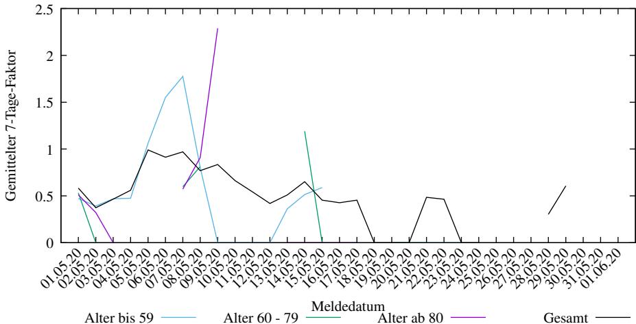
7-Tage-Faktoren der neuen COVID-19 Infizierten in Sachsen-Anhalt (2025-03-09/2005, D. Lippold, https://covid19-de-stats.sourceforge.io/ Lizenz: CC BY-ND 4.0, Daten: Robert Koch-Institut (RKI), dl-de/by-2-0)
