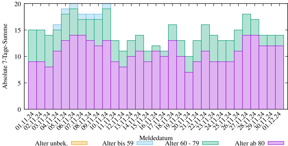
Abs. 7-Tage-Summen der neuen COVID-19 Verstorbenen in Sachsen (2025-03-09/2411, D. Lippold, https://covid19-de-stats.sourceforge.io/ Lizenz: CC BY-ND 4.0, Daten: Robert Koch-Institut (RKI), dl-de/by-2-0)
