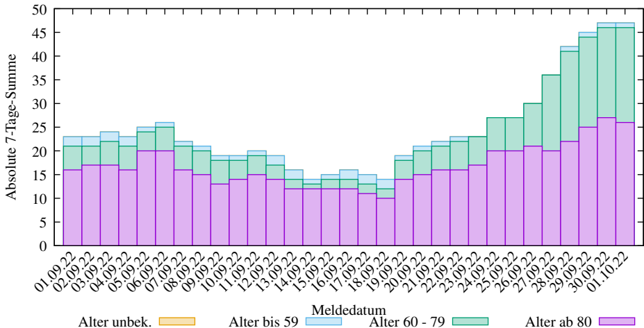
Abs. 7-Tage-Summen der neuen COVID-19 Verstorbenen in Sachsen (2025-03-09/2209, D. Lippold, https://covid19-de-stats.sourceforge.io/ Lizenz: CC BY-ND 4.0, Daten: Robert Koch-Institut (RKI), dl-de/by-2-0)
