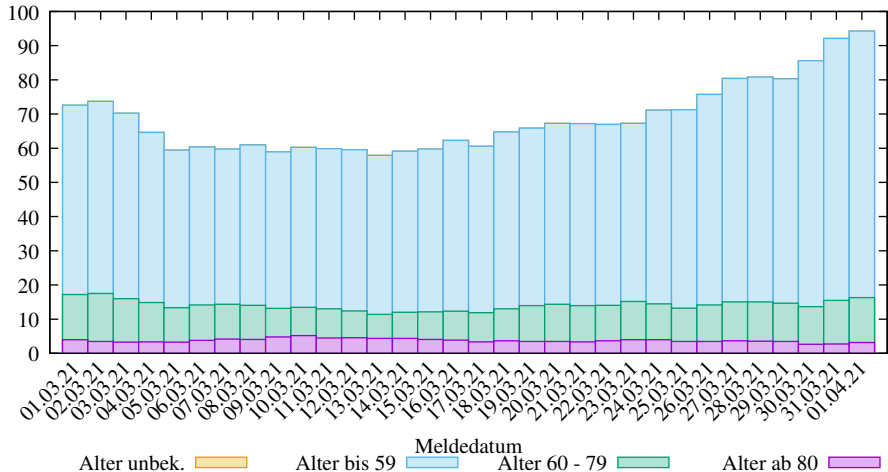
Rel. 7-Tage-Summe der neuen COVID-19 Infizierten in Saarland (2025-03-09/2103, D. Lippold, https://covid19-de-stats.sourceforge.io/ Lizenz: CC BY-ND 4.0, Daten: Robert Koch-Institut (RKI), dl-de/by-2-0)
