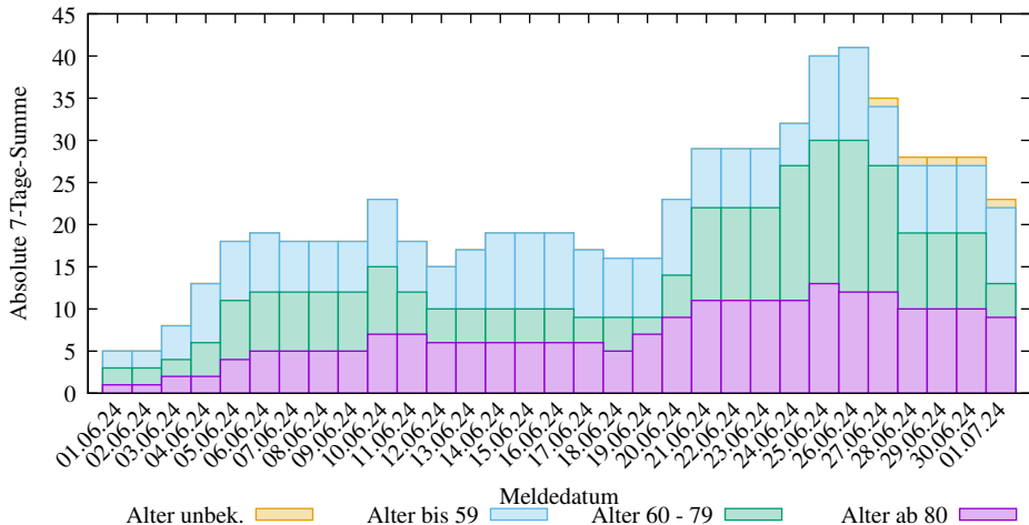
Abs. 7-Tage-Summen der neuen COVID-19 Infizierten in Saarland (2025-03-09/2406, D. Lippold, https://covid19-de-stats.sourceforge.io/ Lizenz: CC BY-ND 4.0, Daten: Robert Koch-Institut (RKI), dl-de/by-2-0)
