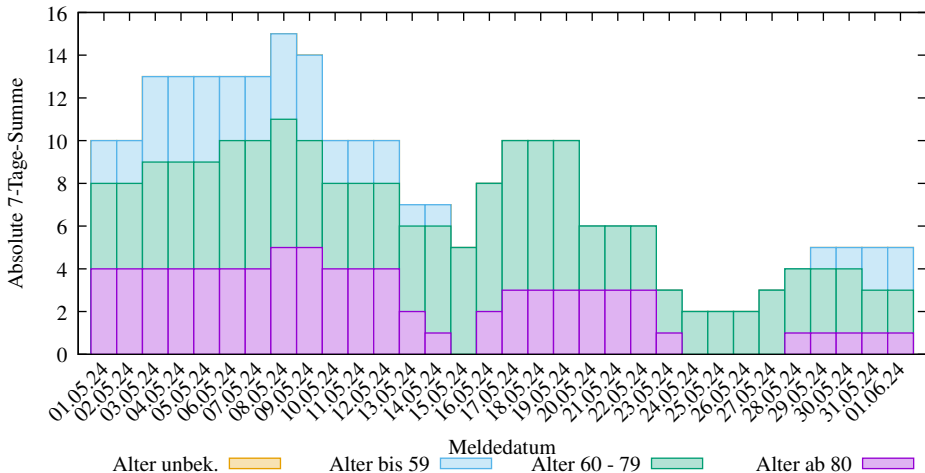
Abs. 7-Tage-Summen der neuen COVID-19 Infizierten in Saarland (2025-03-09/2405, D. Lippold, https://covid19-de-stats.sourceforge.io/ Lizenz: CC BY-ND 4.0, Daten: Robert Koch-Institut (RKI), dl-de/by-2-0)
