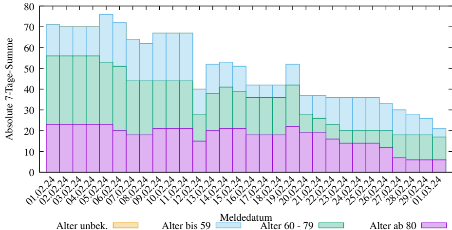
Abs. 7-Tage-Summen der neuen COVID-19 Infizierten in Saarland (2025-07-06/2402, D. Lippold, https://covid19-de-stats.sourceforge.io/ Lizenz: CC BY-ND 4.0, Daten: Robert Koch-Institut (RKI), dl-de/by-2-0)
