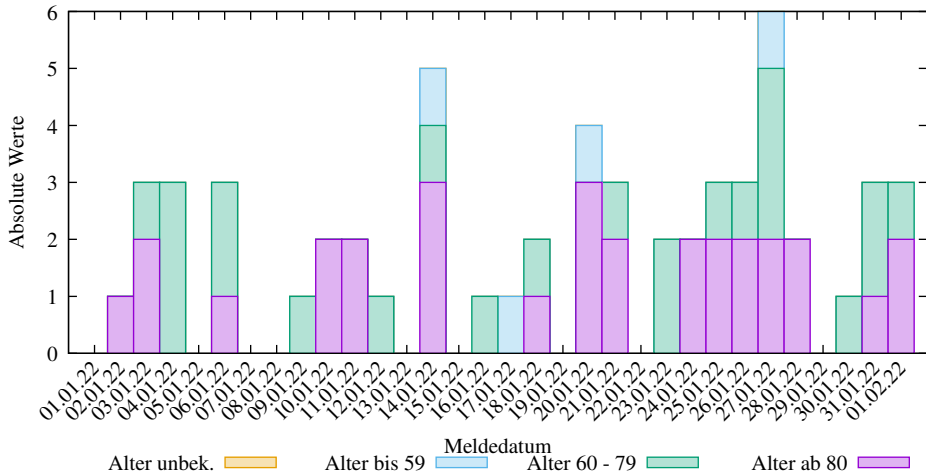
Einzelwerte der neuen COVID-19 Verstorbenen in Saarland (2025-03-09/2201, D. Lippold, https://covid19-de-stats.sourceforge.io/ Lizenz: CC BY-ND 4.0, Daten: Robert Koch-Institut (RKI), dl-de/by-2-0)
