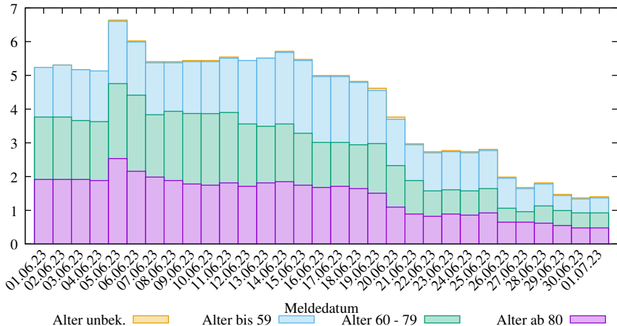
Rel. 7-Tage-Summe der neuen COVID-19 Infizierten in Schleswig-Holstein (2025-07-06/2306, D. Lippold, https://covid19-de-stats.sourceforge.io/ Lizenz: CC BY-ND 4.0, Daten: Robert Koch-Institut (RKI), dl-de/by-2-0)
