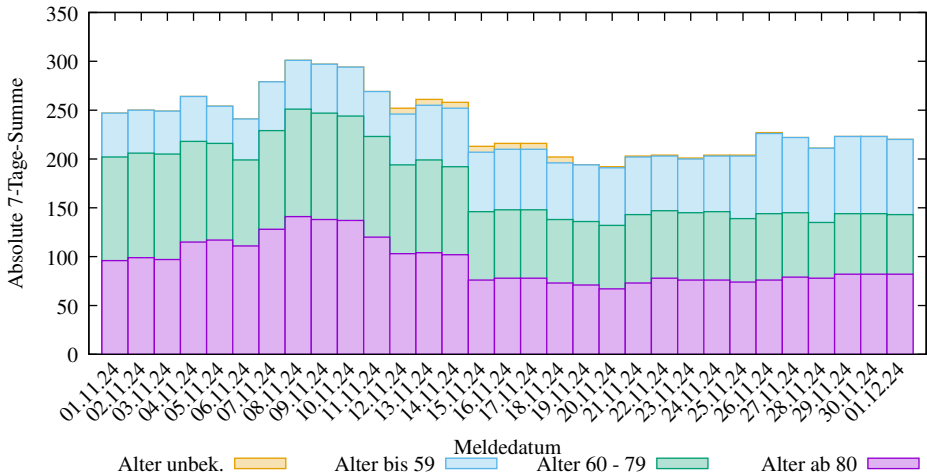
Abs. 7-Tage-Summen der neuen COVID-19 Infizierten in Schleswig-Holstein (2025-03-09/2411, D. Lippold, https://covid19-de-stats.sourceforge.io/ Lizenz: CC BY-ND 4.0, Daten: Robert Koch-Institut (RKI), dl-de/by-2-0)
