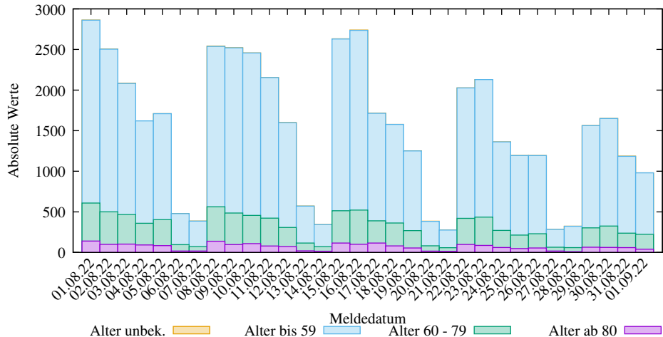
Einzelwerte der neuen COVID-19 Infizierten in Schleswig-Holstein (2025-03-09/2208, D. Lippold, https://covid19-de-stats.sourceforge.io/ Lizenz: CC BY-ND 4.0, Daten: Robert Koch-Institut (RKI), dl-de/by-2-0)
