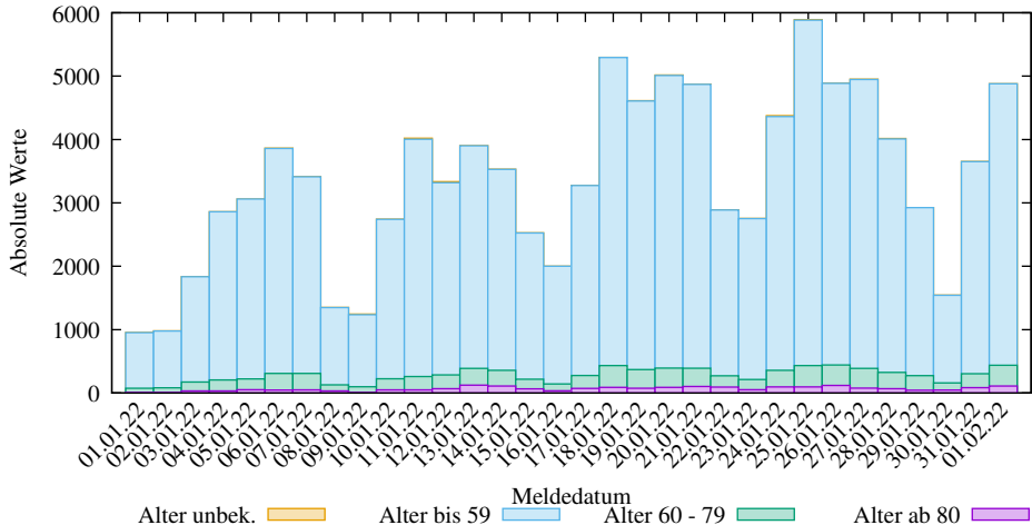
Einzelwerte der neuen COVID-19 Infizierten in Schleswig-Holstein (2025-03-09/2201, D. Lippold, https://covid19-de-stats.sourceforge.io/ Lizenz: CC BY-ND 4.0, Daten: Robert Koch-Institut (RKI), dl-de/by-2-0)
