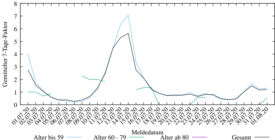
7-Tage-Faktoren der neuen COVID-19 Infizierten in Rheinland-Pfalz (2025-03-09/2007, D. Lippold, https://covid19-de-stats.sourceforge.io/ Lizenz: CC BY-ND 4.0, Daten: Robert Koch-Institut (RKI), dl-de/by-2-0)
