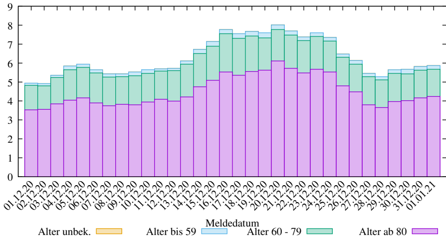
Rel. 7-Tage-Summe der neuen COVID-19 Verstorbenen in Rheinland-Pfalz (2025-03-09/2012, D. Lippold, https://covid19-de-stats.sourceforge.io/ Lizenz: CC BY-ND 4.0, Daten: Robert Koch-Institut (RKI), dl-de/by-2-0)
