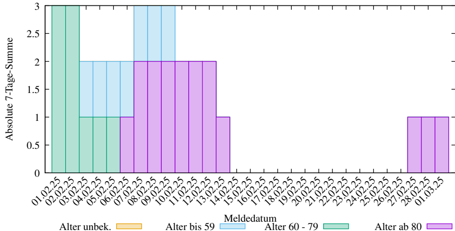
Abs. 7-Tage-Summen der neuen COVID-19 Verstorbenen in Rheinland-Pfalz (2025-04-28/2502, D. Lippold, https://covid19-de-stats.sourceforge.io/ Lizenz: CC BY-ND 4.0, Daten: Robert Koch-Institut (RKI), dl-de/by-2-0)
