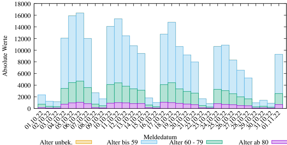
Einzelwerte der neuen COVID-19 Infizierten in Niedersachsen (2025-03-09/2210, D. Lippold, https://covid19-de-stats.sourceforge.io/ Lizenz: CC BY-ND 4.0, Daten: Robert Koch-Institut (RKI), dl-de/by-2-0)
