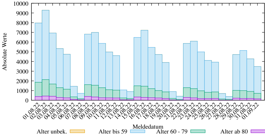
Einzelwerte der neuen COVID-19 Infizierten in Niedersachsen (2025-03-09/2208, D. Lippold, https://covid19-de-stats.sourceforge.io/ Lizenz: CC BY-ND 4.0, Daten: Robert Koch-Institut (RKI), dl-de/by-2-0)
