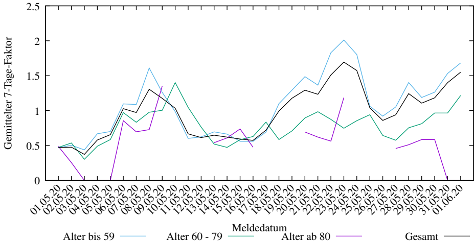
7-Tage-Faktoren der neuen COVID-19 Infizierten in Niedersachsen (2025-03-09/2005, D. Lippold, https://covid19-de-stats.sourceforge.io/ Lizenz: CC BY-ND 4.0, Daten: Robert Koch-Institut (RKI), dl-de/by-2-0)
