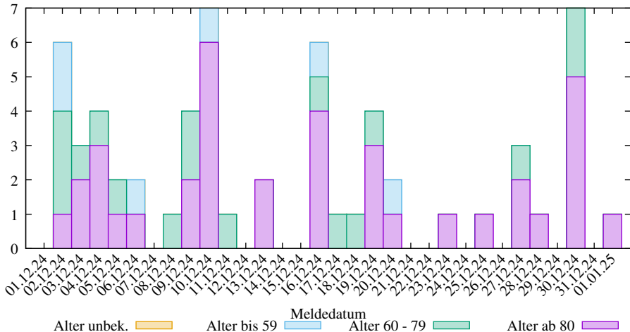
Einzelwerte der neuen COVID-19 Verstorbenen in Niedersachsen (2025-03-09/2412, D. Lippold, https://covid19-de-stats.sourceforge.io/ Lizenz: CC BY-ND 4.0, Daten: Robert Koch-Institut (RKI), dl-de/by-2-0)
