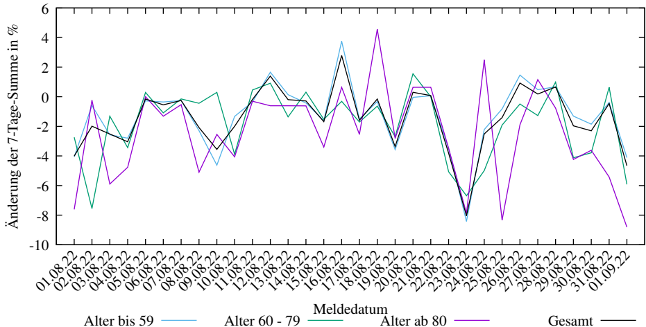
Änderungen der neuen COVID-19 Infizierten in Meckl.-Vorpom. (2025-03-09/2208, D. Lippold, https://covid19-de-stats.sourceforge.io/ Lizenz: CC BY-ND 4.0, Daten: Robert Koch-Institut (RKI), dl-de/by-2-0)
