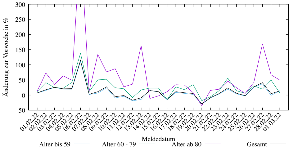
Änderungen der neuen COVID-19 Infizierten in Meckl.-Vorpom. (2025-03-09/2202, D. Lippold, https://covid19-de-stats.sourceforge.io/ Lizenz: CC BY-ND 4.0, Daten: Robert Koch-Institut (RKI), dl-de/by-2-0)
