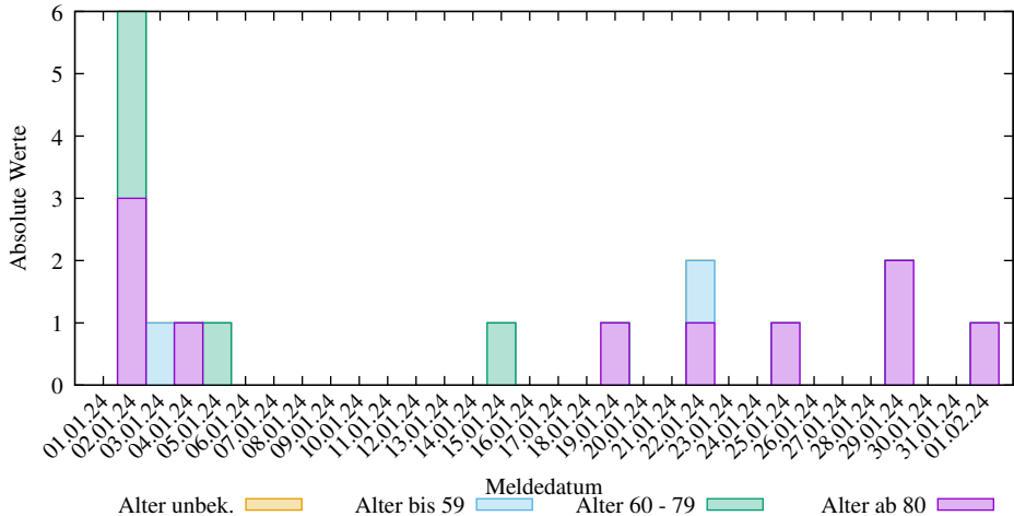
Einzelwerte der neuen COVID-19 Verstorbenen in Meckl.-Vorpom. (2025-03-09/2401, D. Lippold, https://covid19-de-stats.sourceforge.io/ Lizenz: CC BY-ND 4.0, Daten: Robert Koch-Institut (RKI), dl-de/by-2-0)
