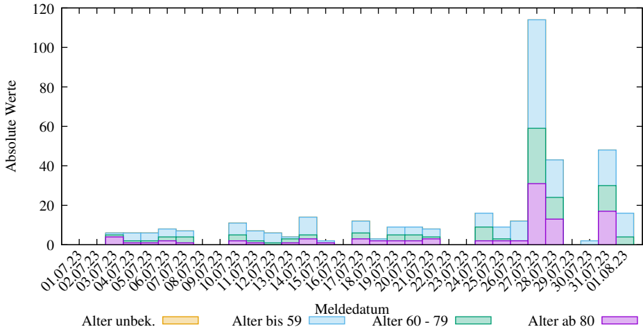
Einzelwerte der neuen COVID-19 Infizierten in Hamburg (2025-03-09/2307, D. Lippold, https://covid19-de-stats.sourceforge.io/ Lizenz: CC BY-ND 4.0, Daten: Robert Koch-Institut (RKI), dl-de/by-2-0)
