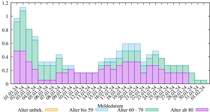
Rel. 7-Tage-Summe der neuen COVID-19 Verstorbenen in Hamburg (2025-03-09/2401, D. Lippold, https://covid19-de-stats.sourceforge.io/ Lizenz: CC BY-ND 4.0, Daten: Robert Koch-Institut (RKI), dl-de/by-2-0)
