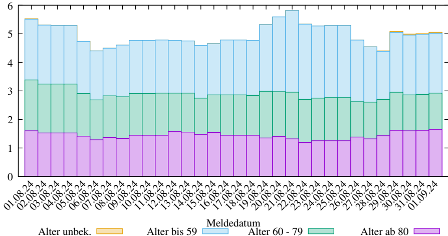
Rel. 7-Tage-Summe der neuen COVID-19 Infizierten in Hessen (2025-03-09/2408, D. Lippold, https://covid19-de-stats.sourceforge.io/ Lizenz: CC BY-ND 4.0, Daten: Robert Koch-Institut (RKI), dl-de/by-2-0)
