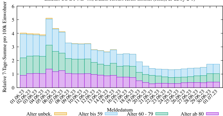
Rel. 7-Tage-Summe der neuen COVID-19 Infizierten in Hessen (2025-03-09/2306, D. Lippold, https://covid19-de-stats.sourceforge.io/ Lizenz: CC BY-ND 4.0, Daten: Robert Koch-Institut (RKI), dl-de/by-2-0)
