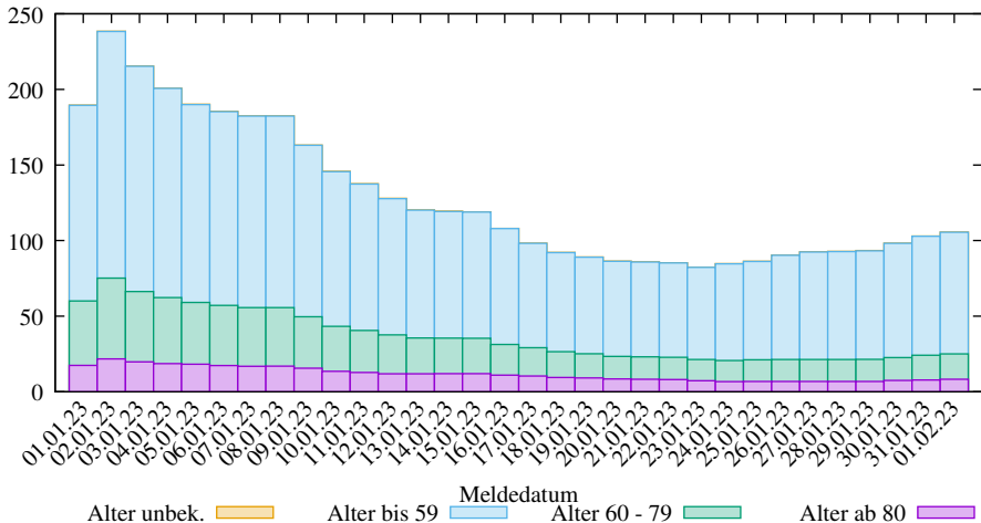
Rel. 7-Tage-Summe der neuen COVID-19 Infizierten in Hessen (2025-03-09/2301, D. Lippold, https://covid19-de-stats.sourceforge.io/ Lizenz: CC BY-ND 4.0, Daten: Robert Koch-Institut (RKI), dl-de/by-2-0)
