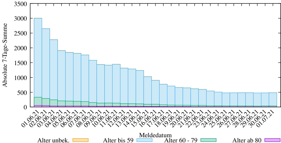
Abs. 7-Tage-Summen der neuen COVID-19 Infizierten in Hessen (2025-03-09/2106, D. Lippold, https://covid19-de-stats.sourceforge.io/ Lizenz: CC BY-ND 4.0, Daten: Robert Koch-Institut (RKI), dl-de/by-2-0)
