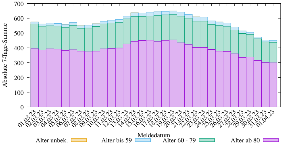
Abs. 7-Tage-Summen der neuen COVID-19 Verstorbenen in Deutschland gesamt (2025-03-09/2303, D. Lippold, https://covid19-de-stats.sourceforge.io/ Lizenz: CC BY-ND 4.0, Daten: Robert Koch-Institut (RKI), dl-de/by-2-0)
