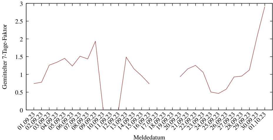
7-Tage-Faktoren der neuen COVID-19 Verstorbenen in Deutschland gesamt (2025-03-09/2309, D. Lippold, https://covid19-de-stats.sourceforge.io/ Lizenz: CC BY-ND 4.0, Daten: Robert Koch-Institut (RKI), dl-de/by-2-0)
