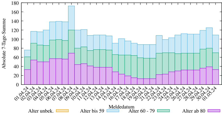
Abs. 7-Tage-Summen der neuen COVID-19 Infizierten in Bayern (2025-03-09/2404, D. Lippold, https://covid19-de-stats.sourceforge.io/ Lizenz: CC BY-ND 4.0, Daten: Robert Koch-Institut (RKI), dl-de/by-2-0)
