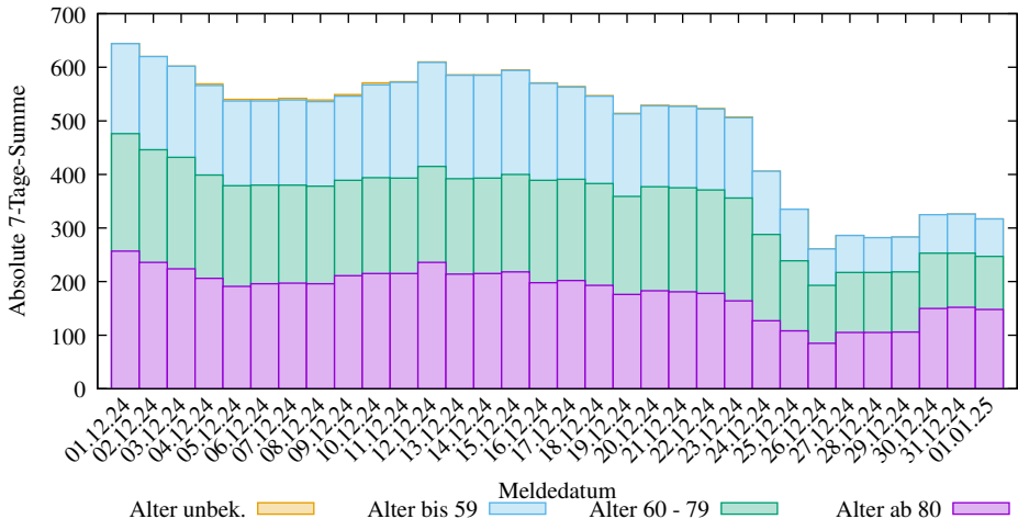
Abs. 7-Tage-Summen der neuen COVID-19 Infizierten in Baden-Württemberg (2025-03-09/2412, D. Lippold, https://covid19-de-stats.sourceforge.io/ Lizenz: CC BY-ND 4.0, Daten: Robert Koch-Institut (RKI), dl-de/by-2-0)
