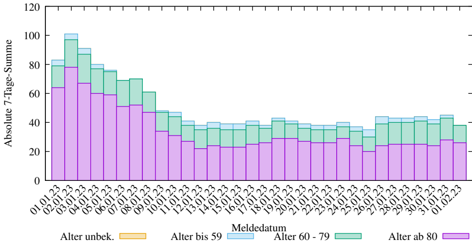
Abs. 7-Tage-Summen der neuen COVID-19 Verstorbenen in Baden-Württemberg (2025-03-09/2301, D. Lippold, https://covid19-de-stats.sourceforge.io/ Lizenz: CC BY-ND 4.0, Daten: Robert Koch-Institut (RKI), dl-de/by-2-0)
