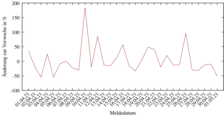
Änderungen der neuen COVID-19 Verstorbenen in Baden-Württemberg (2025-03-09/2104, D. Lippold, https://covid19-de-stats.sourceforge.io/ Lizenz: CC BY-ND 4.0, Daten: Robert Koch-Institut (RKI), dl-de/by-2-0)
