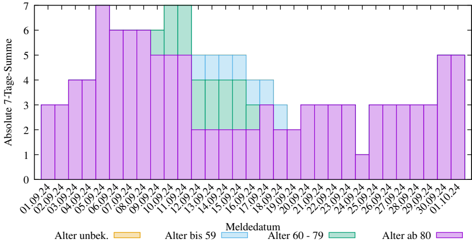
Abs. 7-Tage-Summen der neuen COVID-19 Verstorbenen in Berlin (2025-03-09/2409, D. Lippold, https://covid19-de-stats.sourceforge.io/ Lizenz: CC BY-ND 4.0, Daten: Robert Koch-Institut (RKI), dl-de/by-2-0)
