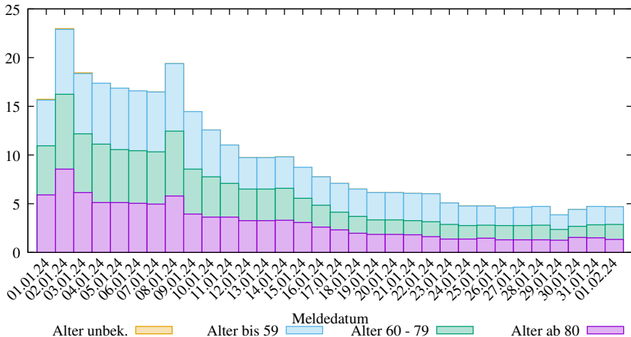
Rel. 7-Tage-Summe der neuen COVID-19 Infizierten in Brandenburg (2025-03-09/2401, D. Lippold, https://covid19-de-stats.sourceforge.io/ Lizenz: CC BY-ND 4.0, Daten: Robert Koch-Institut (RKI), dl-de/by-2-0)
