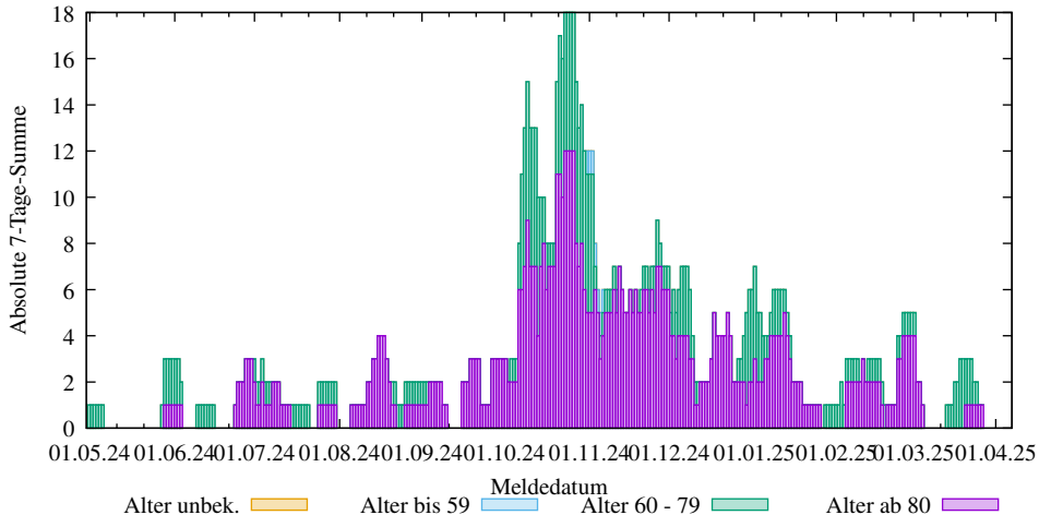
Abs. 7-Tage-Summen der neuen COVID-19 Verstorbenen in Brandenburg (2025-04-28/Short, D. Lippold, https://covid19-de-stats.sourceforge.io/ Lizenz: CC BY-ND 4.0, Daten: Robert Koch-Institut (RKI), dl-de/by-2-0)
