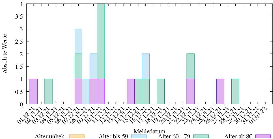
Einzelwerte der neuen COVID-19 Verstorbenen in SK Wiesbaden (2025-07-06/2112, D. Lippold, https://covid19-de-stats.sourceforge.io/ Lizenz: CC BY-ND 4.0, Daten: Robert Koch-Institut (RKI), dl-de/by-2-0)
