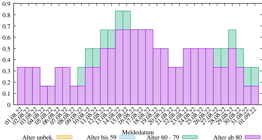
Rel. 7-Tage-Summe der neuen COVID-19 Verstorbenen in LK Rhein-Sieg-Kreis (2025-07-06/2208, D. Lippold, https://covid19-de-stats.sourceforge.io/ ) Lizenz: CC BY-ND 4.0, Daten: Robert Koch-Institut (RKI), dl-de/by-2-0)
