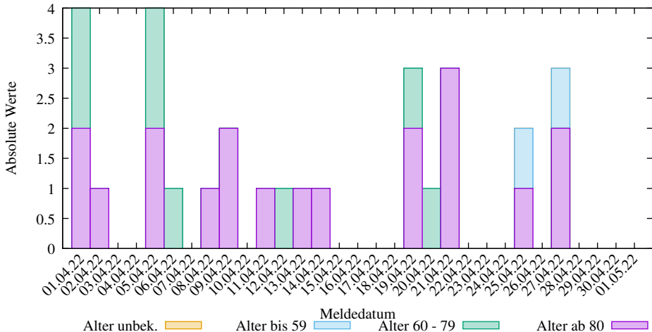
Einzelwerte der neuen COVID-19 Verstorbenen in LK Regv. Saarbrücken (2025-03-09/2204, D. Lippold, https://covid19-de-stats.sourceforge.io/ Lizenz: CC BY-ND 4.0, Daten: Robert Koch-Institut (RKI), dl-de/by-2-0)
