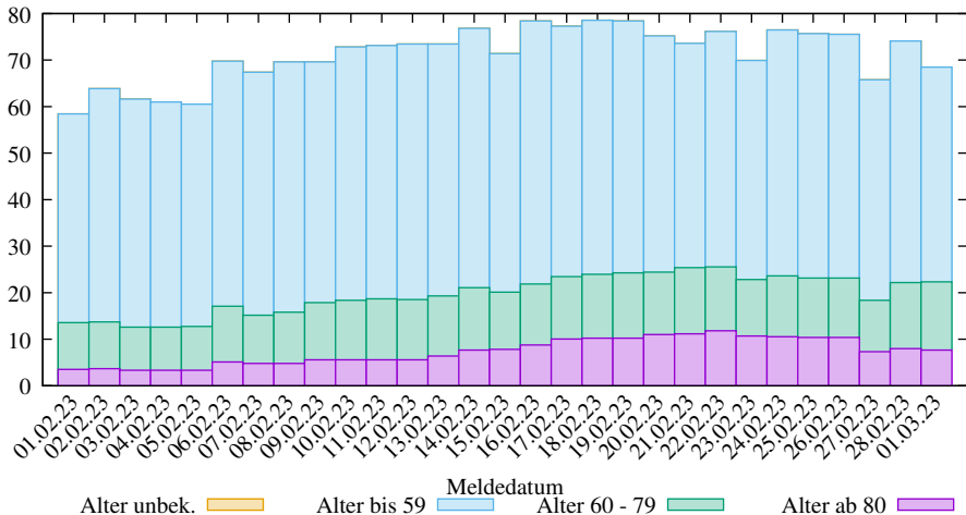
Rel. 7-Tage-Summe der neuen COVID-19 Infizierten in SK Stuttgart (2025-03-09/2302, D. Lippold, https://covid19-de-stats.sourceforge.io/ Lizenz: CC BY-ND 4.0, Daten: Robert Koch-Institut (RKI), dl-de/by-2-0)
