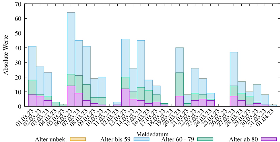
Einzelwerte der neuen COVID-19 Infizierten in SK Stuttgart (2025-03-09/2303, D. Lippold, https://covid19-de-stats.sourceforge.io/ Lizenz: CC BY-ND 4.0, Daten: Robert Koch-Institut (RKI), dl-de/by-2-0)
