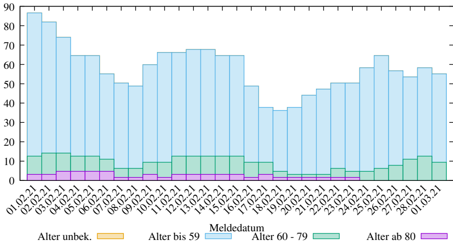
Rel. 7-Tage-Summe der neuen COVID-19 Infizierten in SK Rosenheim (2025-03-09/2102, D. Lippold, https://covid19-de-stats.sourceforge.io/ Lizenz: CC BY-ND 4.0, Daten: Robert Koch-Institut (RKI), dl-de/by-2-0)
