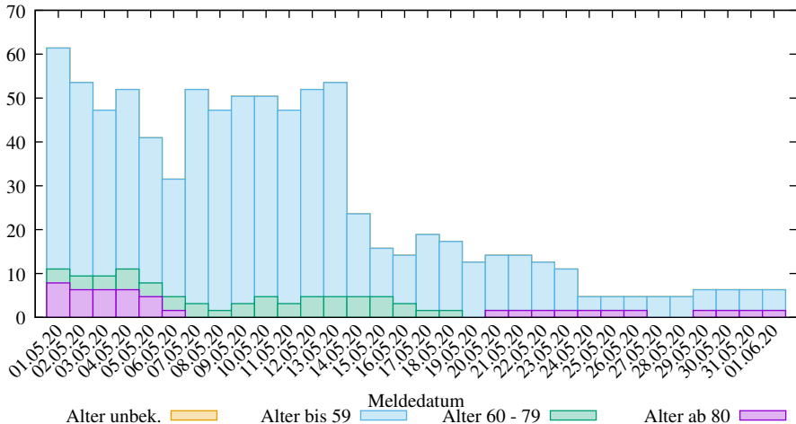
Rel. 7-Tage-Summe der neuen COVID-19 Infizierten in SK Rosenheim (2025-03-09/2005, D. Lippold, https://covid19-de-stats.sourceforge.io/ Lizenz: CC BY-ND 4.0, Daten: Robert Koch-Institut (RKI), dl-de/by-2-0)
