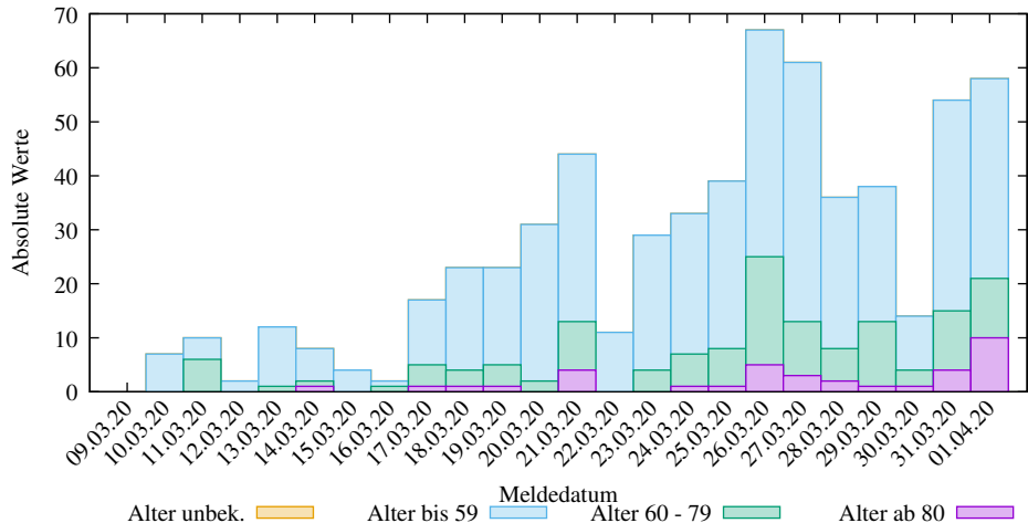
Einzelwerte der neuen COVID-19 Infizierten in LK Rems-Murr-Kreis (2025-03-09/2003, D. Lippold, https://covid19-de-stats.sourceforge.io/ Lizenz: CC BY-ND 4.0, Daten: Robert Koch-Institut (RKI), dl-de/by-2-0)
