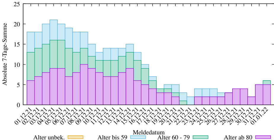
Abs. 7-Tage-Summen der neuen COVID-19 Verstorbenen in LK Rems-Murr-Kreis (2025-03-09/2112, D. Lippold, https://covid19-de-stats.sourceforge.io/ Lizenz: CC BY-ND 4.0, Daten: Robert Koch-Institut (RKI), dl-de/by-2-0)
