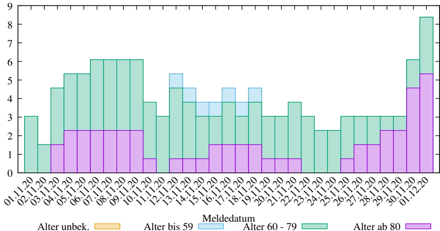
Rel. 7-Tage-Summe der neuen COVID-19 Verstorbenen in SK Offenbach (2025-03-09/2011, D. Lippold, https://covid19-de-stats.sourceforge.io/ Lizenz: CC BY-ND 4.0, Daten: Robert Koch-Institut (RKI), dl-de/by-2-0)
