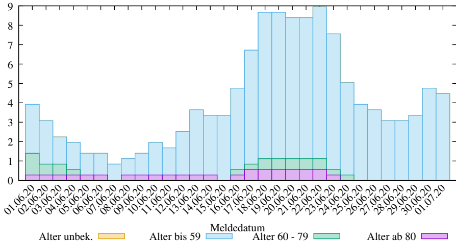
Rel. 7-Tage-Summe der neuen COVID-19 Infizierten in LK Offenbach (2025-03-09/2006, D. Lippold, https://covid19-de-stats.sourceforge.io/ Lizenz: CC BY-ND 4.0, Daten: Robert Koch-Institut (RKI), dl-de/by-2-0)
